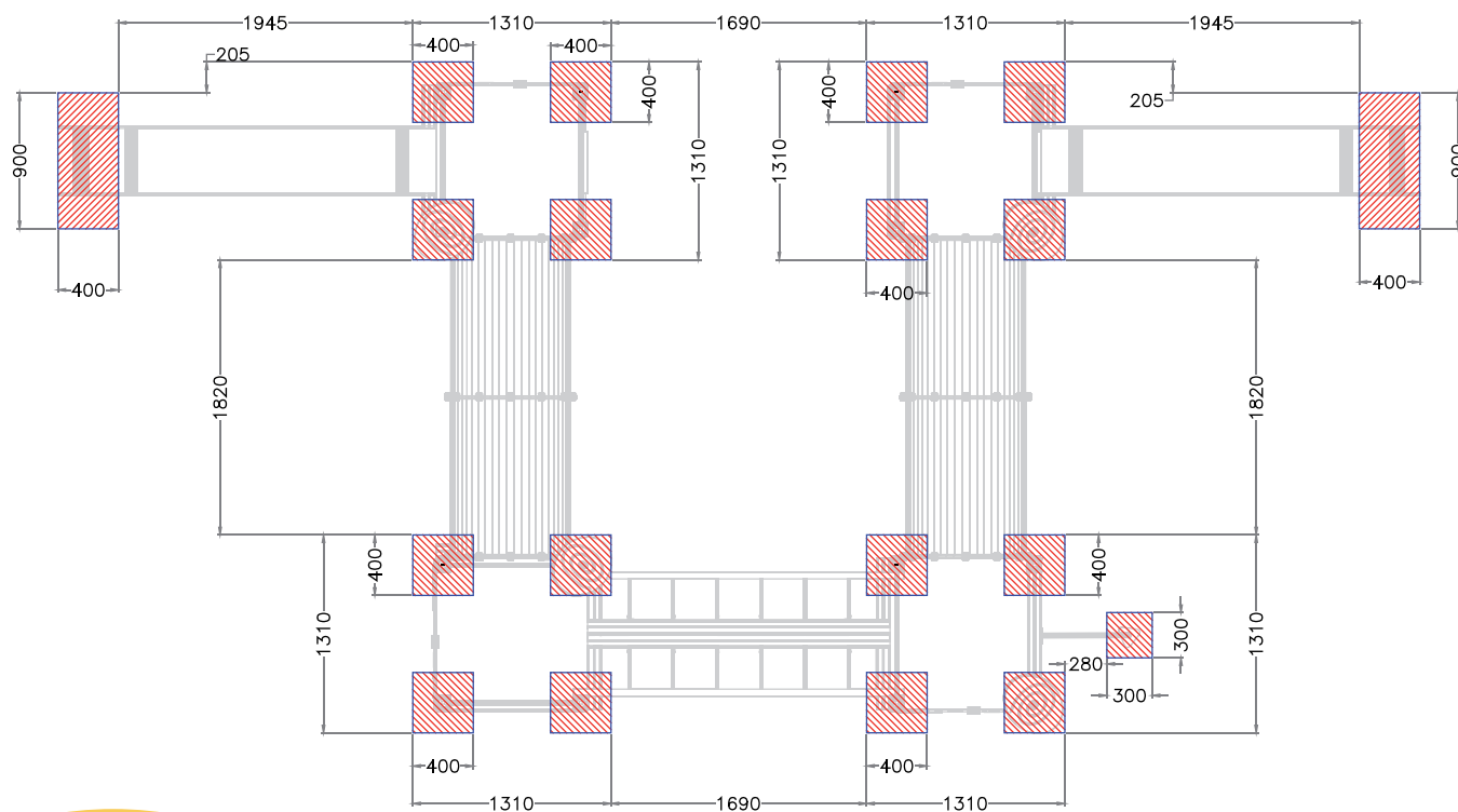
PLANTA CIMENTACION
