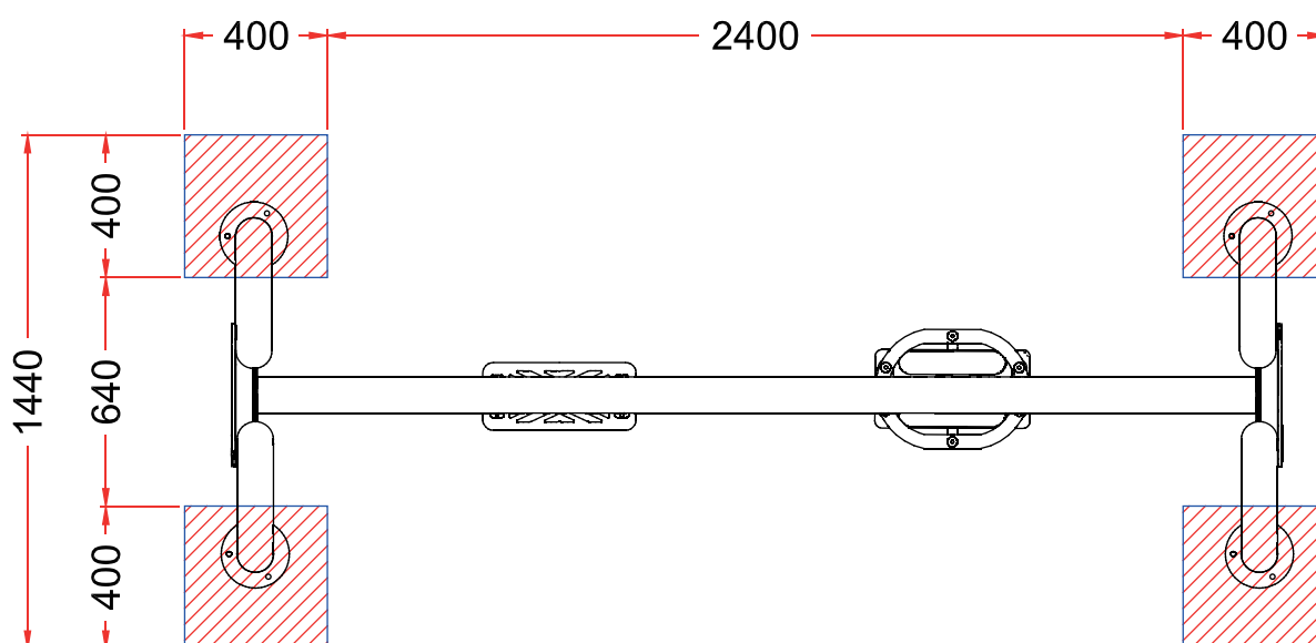
PLANTA CIMENTACION
