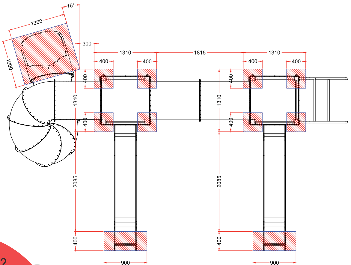
PLANTA CIMENTACION
