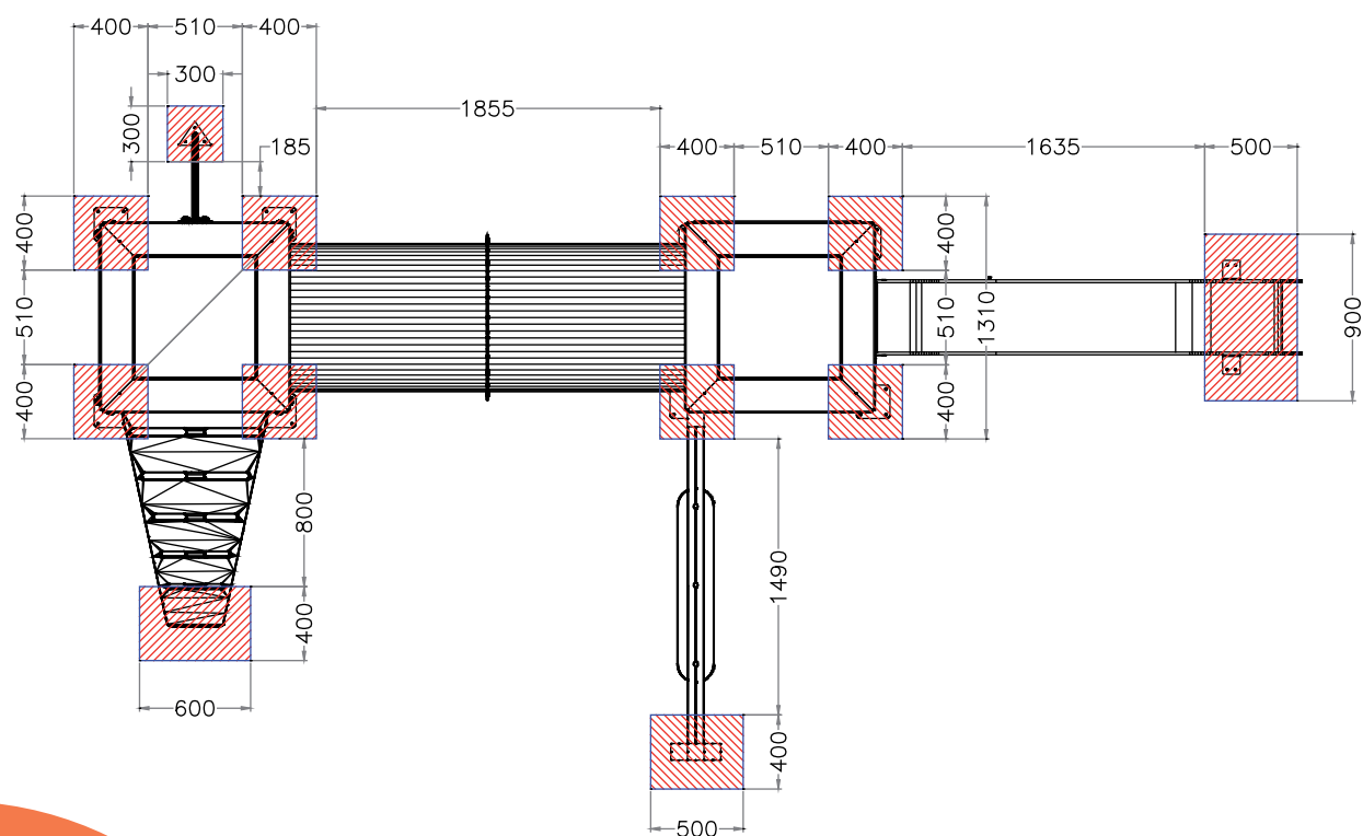
PLANTA CIMENTACION
