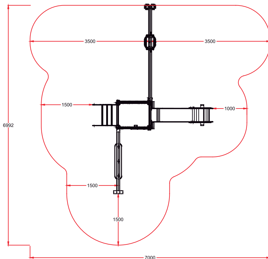
PLANTA
